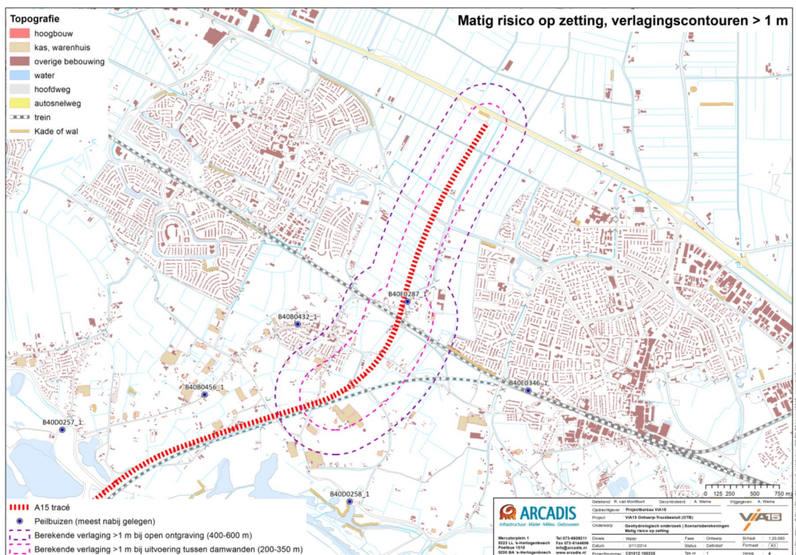
Figuur 7.2 Overzicht van matig risico op zetting langs het wegtracé o.b.v de berekende grondwaterstand-verlaging van meer dan 1 m voor uitvoering in 'open ontgraving' (worst case; paarse onderbroken lijn) en uitvoering tussen damwanden (roze onderbroken lijn).
